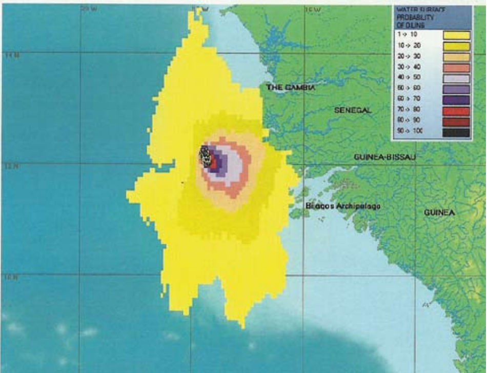
: En cas de pollution accidentelle, la nappe de pétrole dérive selon une direction qui dépend des vents et des courants (probabilité d'une pollution de surface en cas d'accident sur le site de forage Kora)
